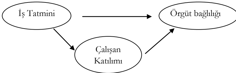
Şekil 1: Kavramsal Model
