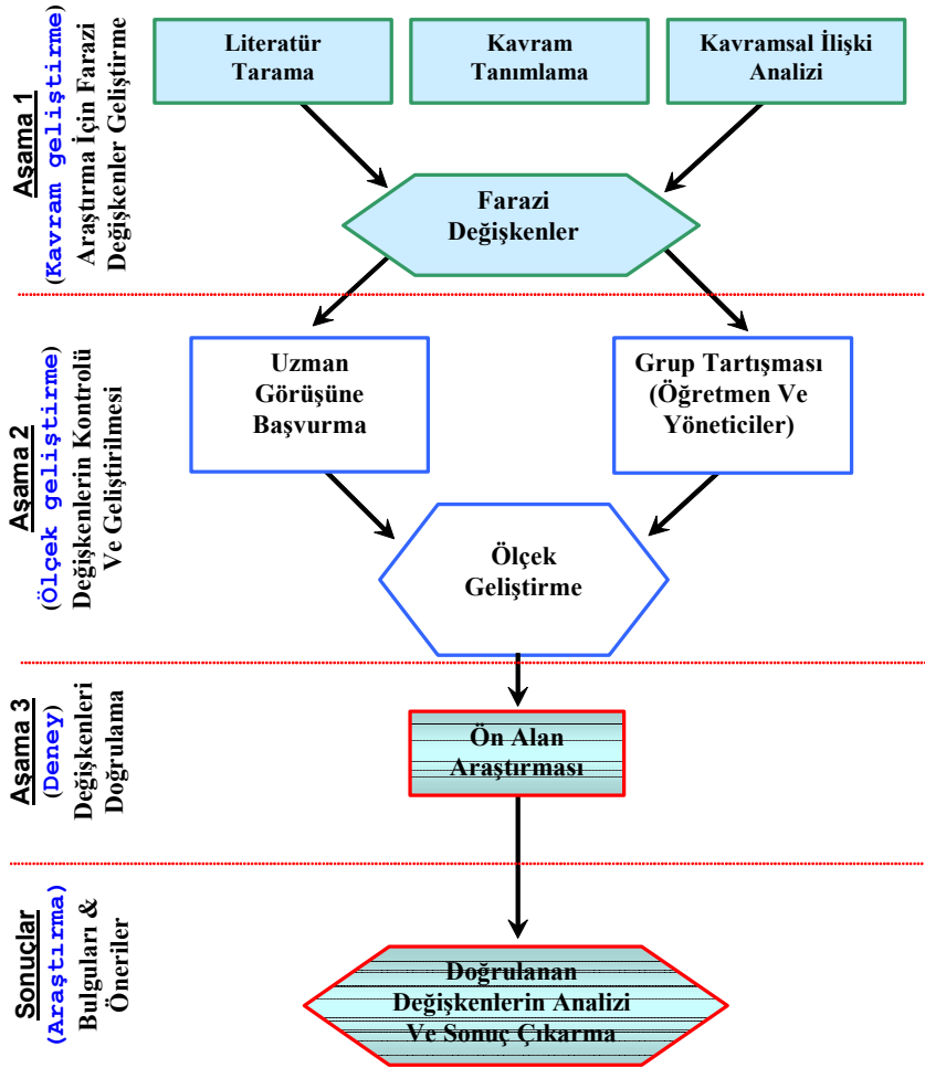
Şekil 1 Araştırmanın tasarımı
