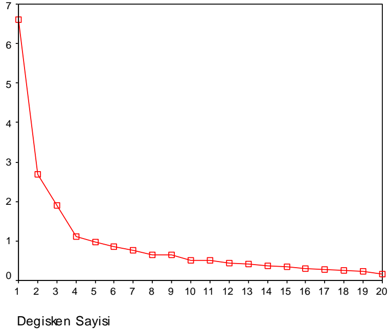
Şekil 1: Özdeğerlerin Dağılımı
