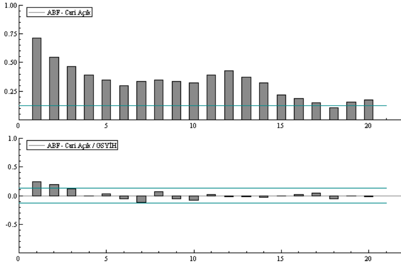
Grafik 1. Cari Açığın ve Cari Açığın GSYİH'ye Oranının Ardışık Bağlanım Fonksiyonlarının Bağım Çizimleri
