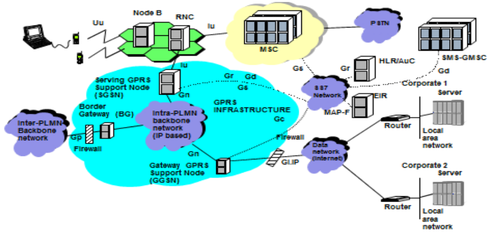
Şekil 1 - UMTS Şebeke Mimarisi
