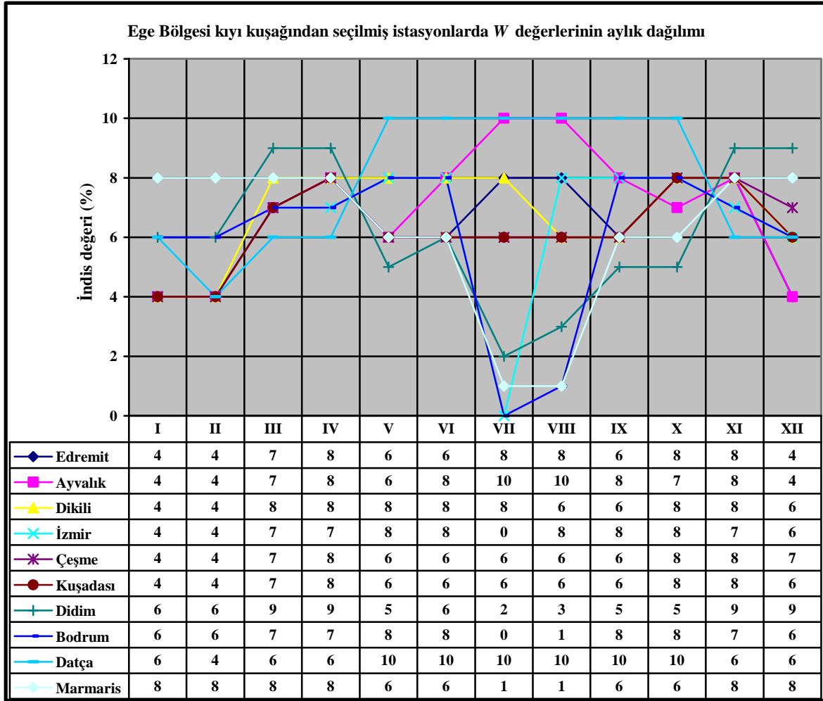
Şekil 4. Ege Bölgesi kıyı kuşağında seçilmiş istasyonlarda W değerlerinin aylık dağılımı (1975-2008 dönemi)
