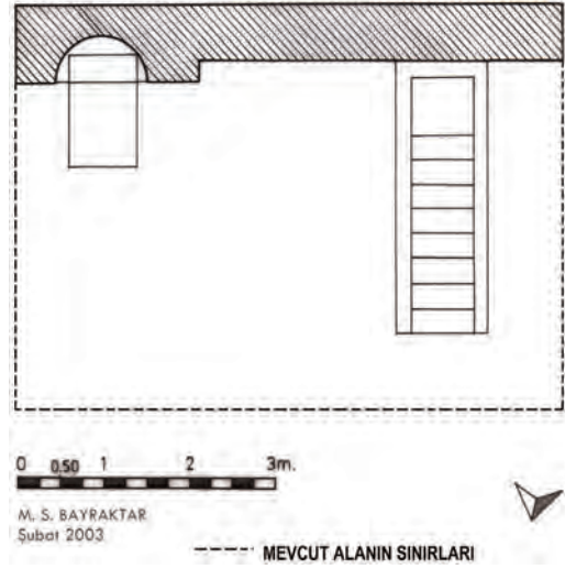
Şekil 3 Veziroköprü Köprülü Mehmed Paşa Namazgâhı Planı. (2008 Restorasyonu Öncesi Durumu).
