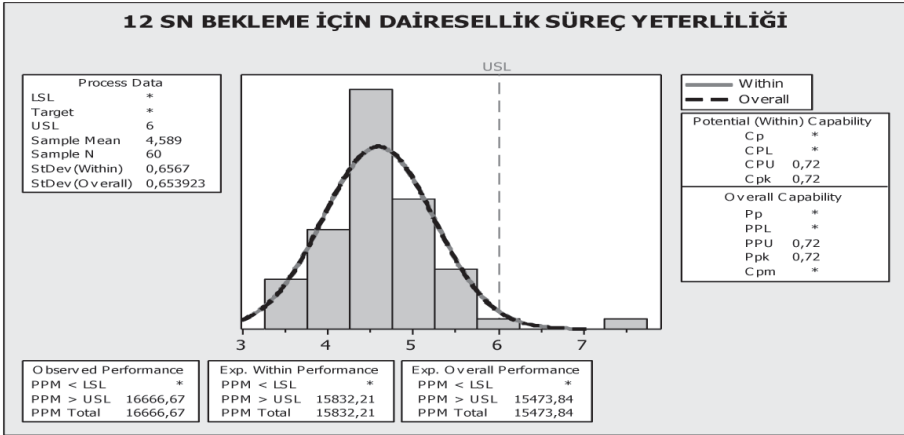
Şekil 9. 12 sn Bekleme İçin Dairesellik Süreç Yeterliliği Grafiği
