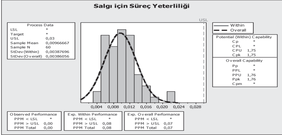
Şekil 10 . Salgı İçin Süreç Yeterliliği
