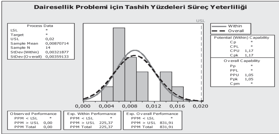
Şekil 12. İyileştirme Sonrası Dairesellik ve Salgı Problemi İçin Tashih Yüzdeleri Süreç Yeterliliği
