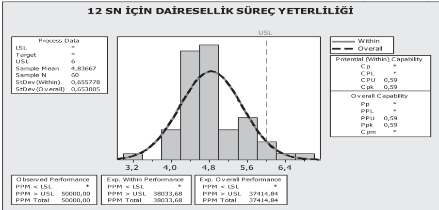
Şekil 8. 12 sn İçin Dairesellik Süreç Yeterliliği Grafği
