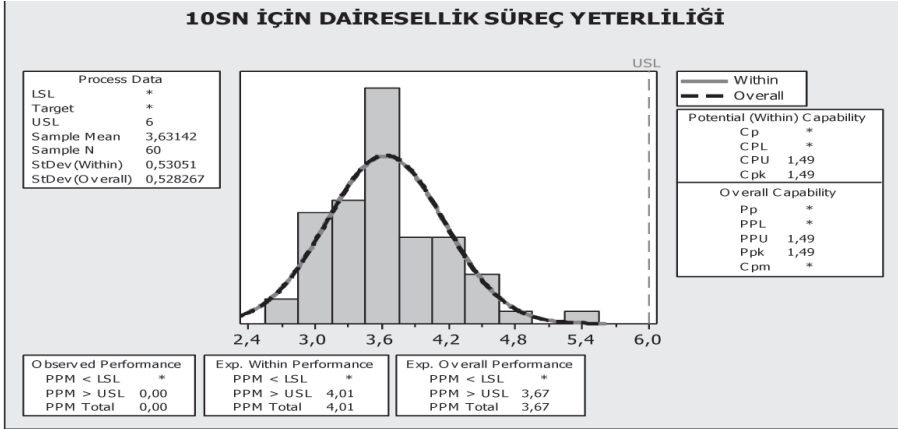
Şekil 7. 10 sn İçin Dairesellik Süreç Yeterliliği Grafği
