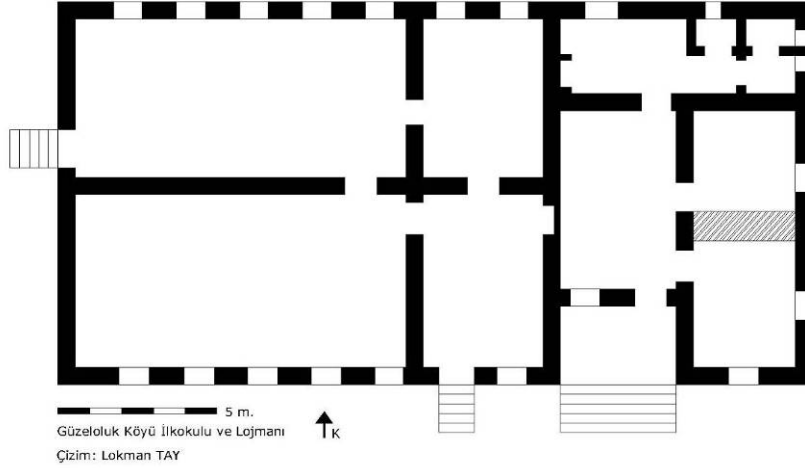
Çizim-4: İlkokul ve lojmanın planı.
