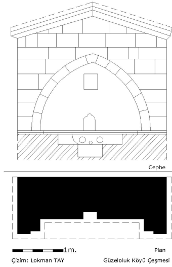
Çizim-3: Çeşmenin planı ve cephe görünüşü.
