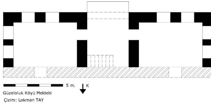
Çizim-1: Mektebin ikinci kat planı.
