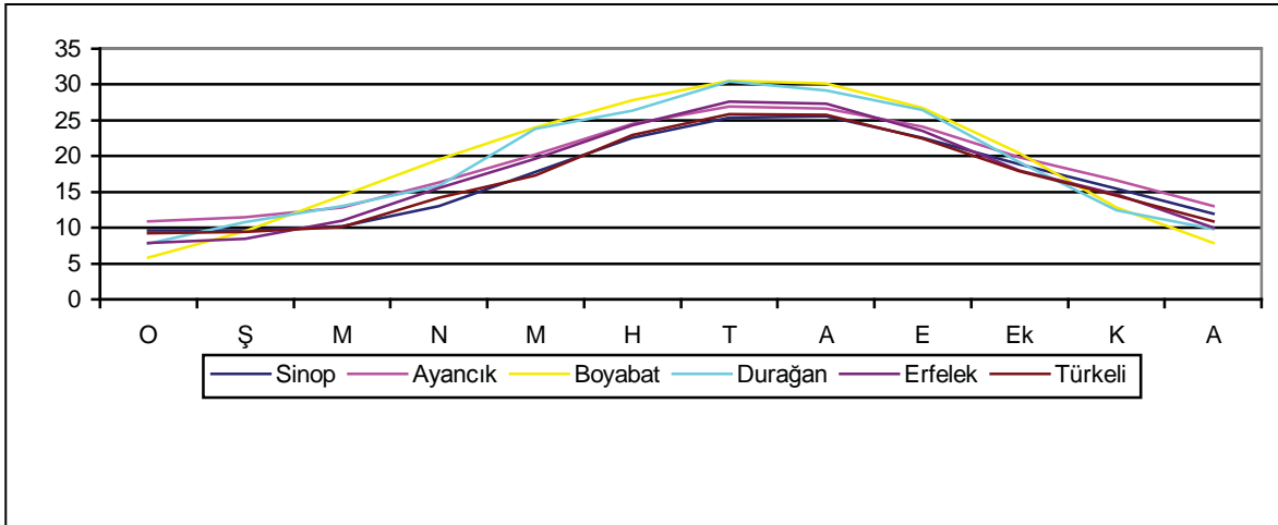
Şekil 19. Sinop'taki meteoroloji istasyonlarında maksimum sıcaklıkların aylara dağılımı (°C).
