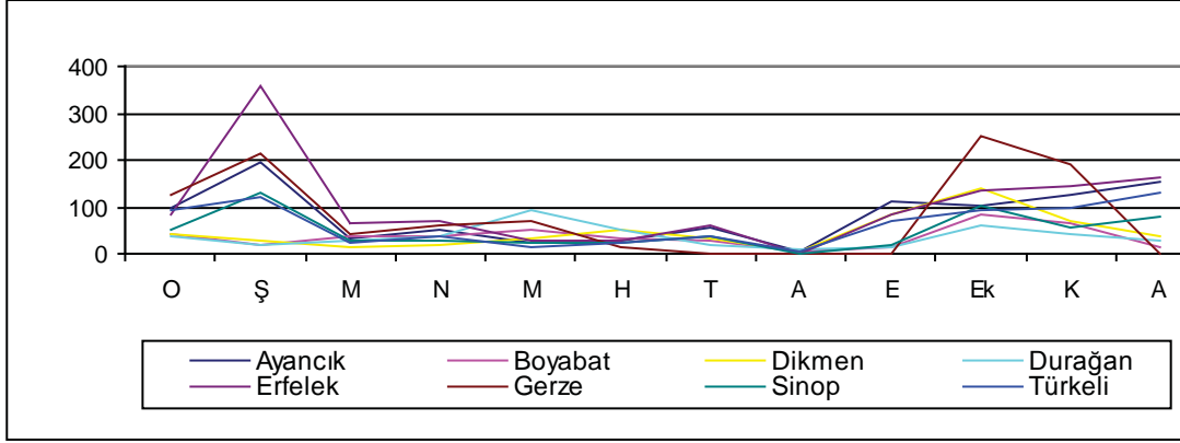
Şekil 14. Sinop ilindeki meteoroloji istasyonlarında 1985 yılı aylık toplam yağış miktarları (mm).
