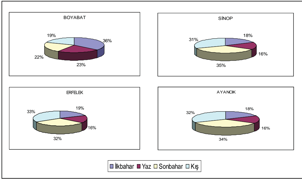
Şekil 8. Sinop-Boyabat-Ayancık-Erfelek istasyonlarında yağışın mevsimlere dağılımı (%).
