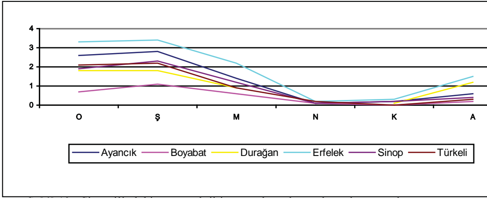
Şekil 10. Sinop ilindeki meteoroloji istasyonlarında ortalama kar yağışlı gün sayısı.
