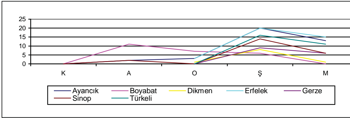
Şekil 16. Sinop'taki Meteoroloji İstasyonlarında 1984-1985 Kış Mevsimi Karla Örtülü Günler Sayısı.
