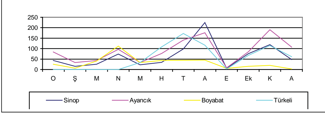
Şekil 13. Sinop, Ayancık, Boyabat ve Türkeli istasyonlarında 1984 yılı aylık toplam yağış miktarları (mm).
