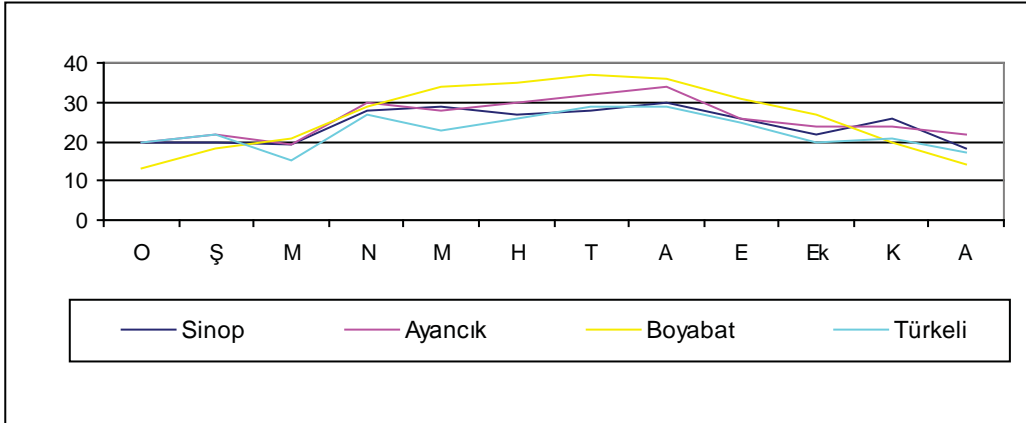
Şekil 22. Sinop, Ayancık, Boyabat ve Türkeli İstasyonlarında 1985 Yılı Maksimum Sıcaklıklar (°C).
