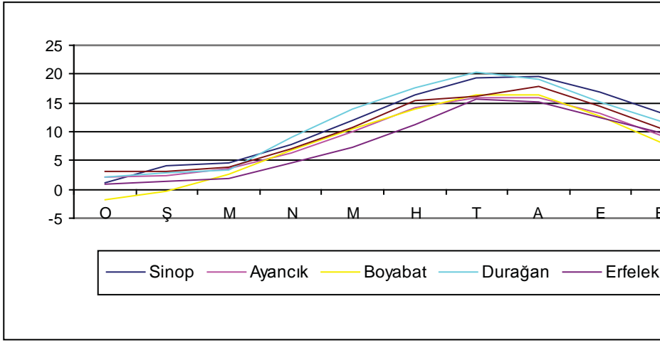
Şekil 20. Sinop'taki meteoroloji istasyonlarında minimum sıcaklıkların aylara dağılımı (°C).
