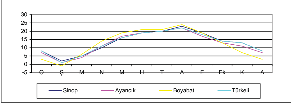
Şekil 21. Sinop, Ayancık, Boyabat ve Türkeli İstasyonlarında 1985 Yılı Aylık Ortalama Sıcaklıklar (°C).
