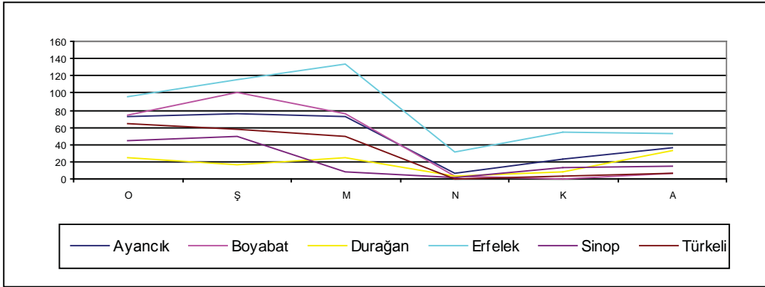
Şekil 12. Sinop ilindeki meteoroloji istasyonlarında en yüksek kar örtüsü kalınlığı (cm).
